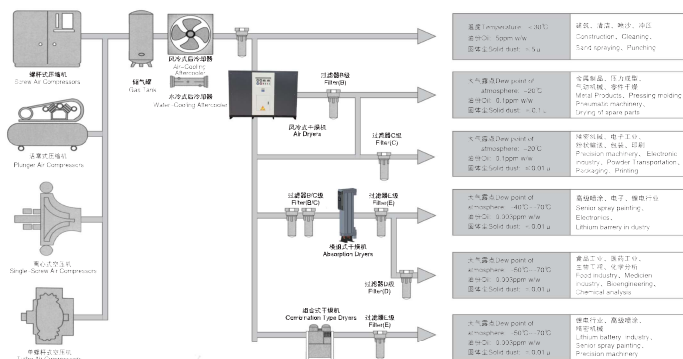
连接示意图 Connection Diagram
